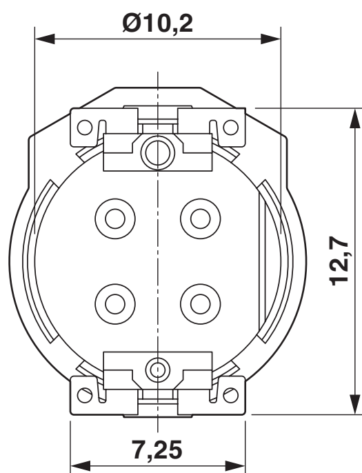
Rysunek wymiarowy
