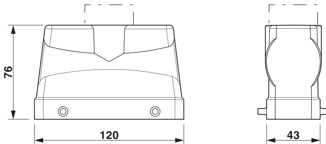
Rysunek wymiarowy
