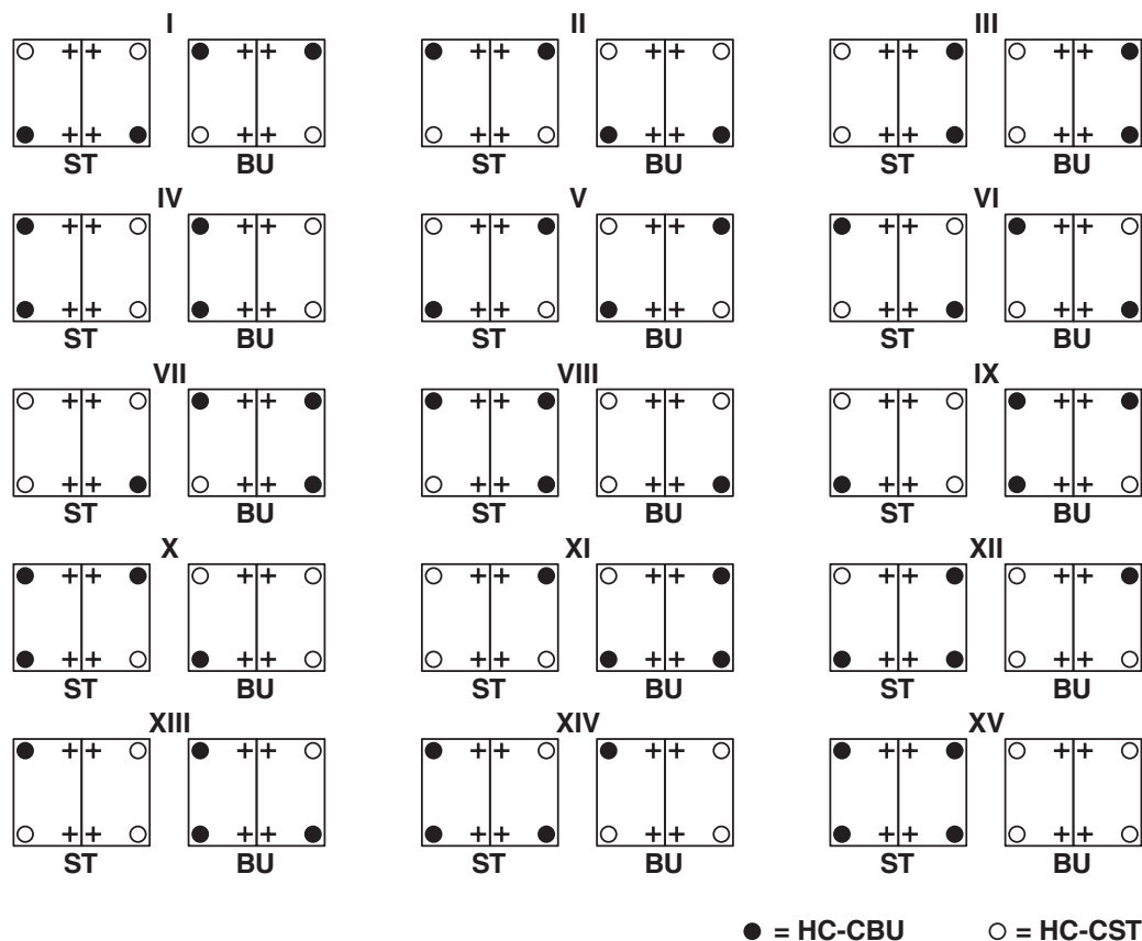
Rysunek schematyczny
