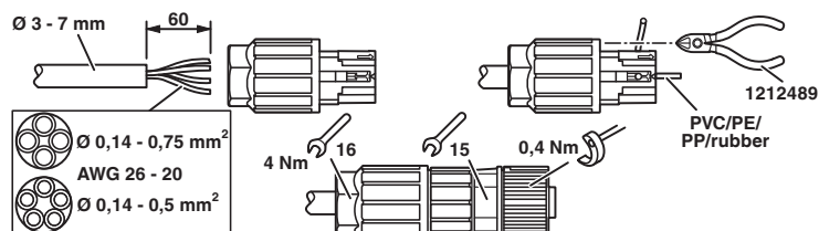
rysunek funkcyjny
