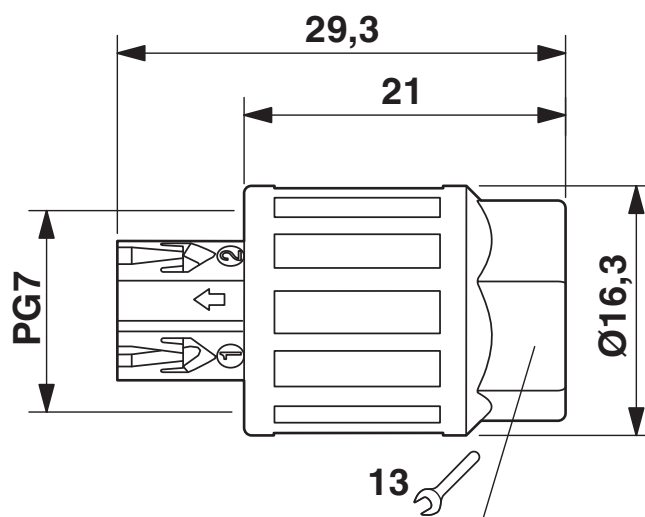
Rysunek wymiarowy
