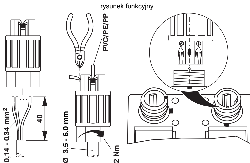
Rysunek schematyczny
