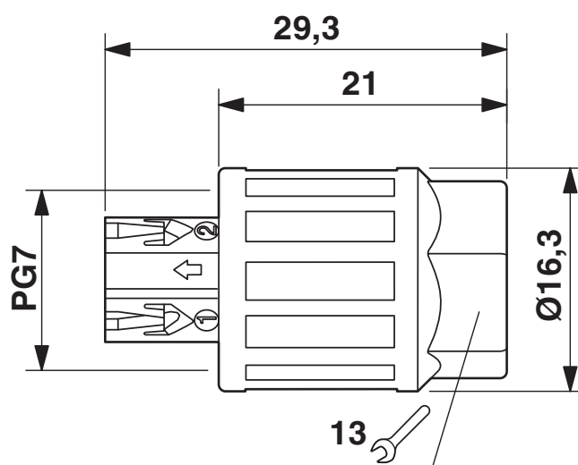
Rysunek wymiarowy
