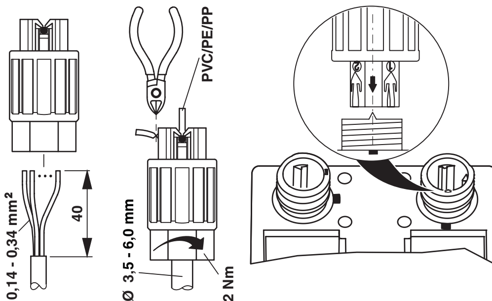
rysunek funkcyjny
