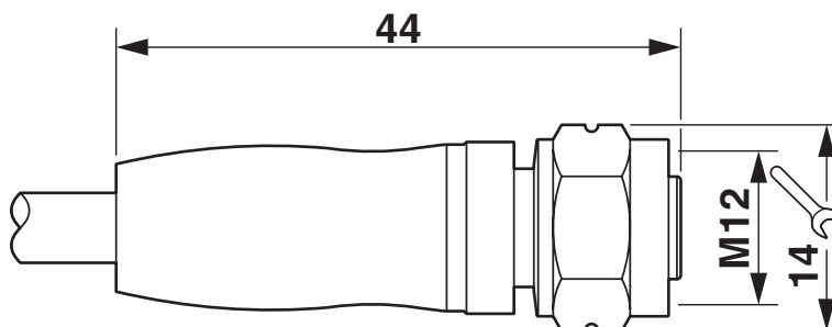
Rysunek wymiarowy
