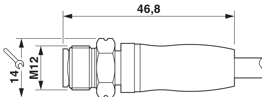
Rysunek wymiarowy
