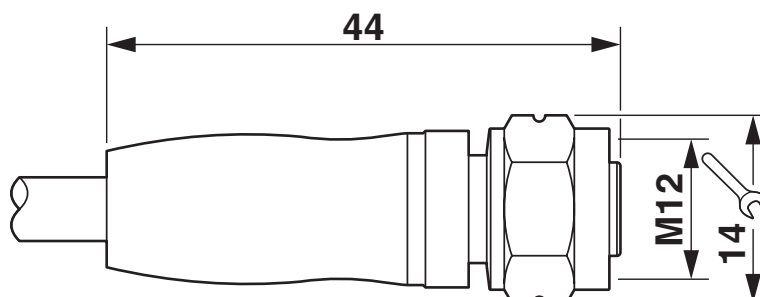
Rysunek wymiarowy
