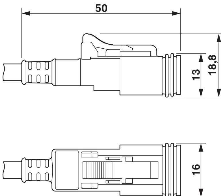
Rysunek wymiarowy
