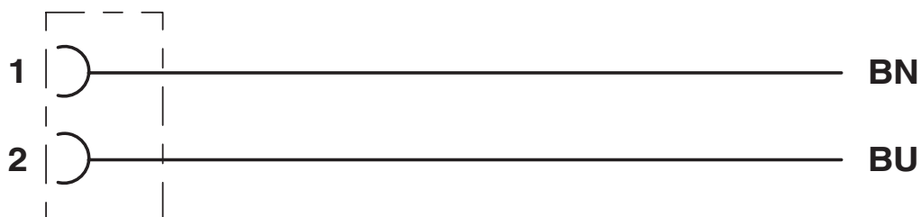
Schemat
