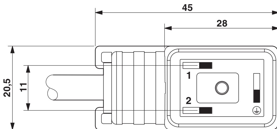
Wtyk zaworowy typ BI
