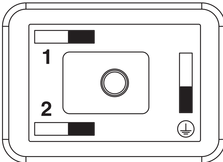
Układ styków wtyk zaworowy, typ BI
