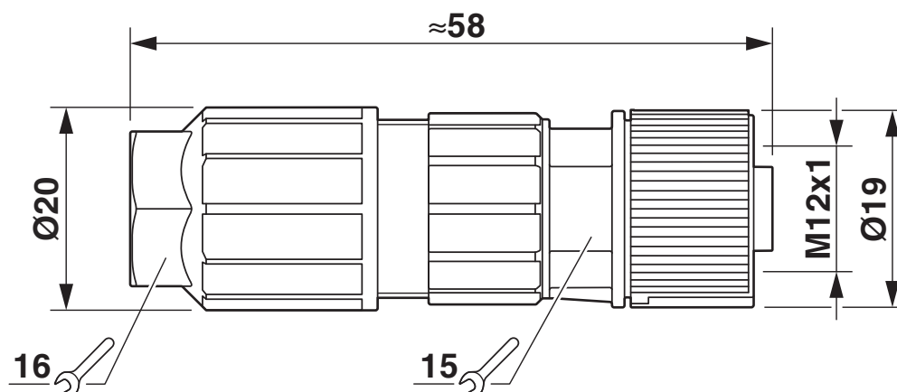
Rysunek wymiarowy
