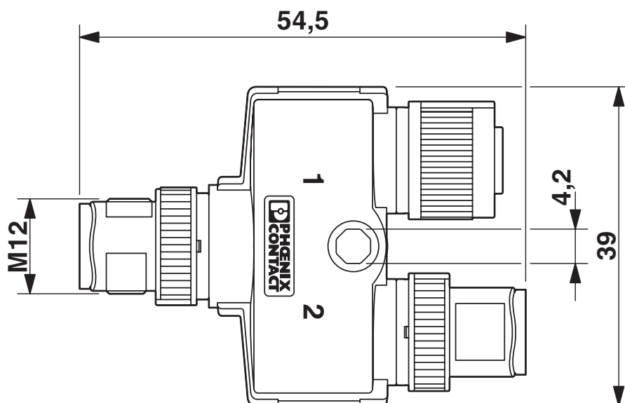
Rysunek wymiarowy
