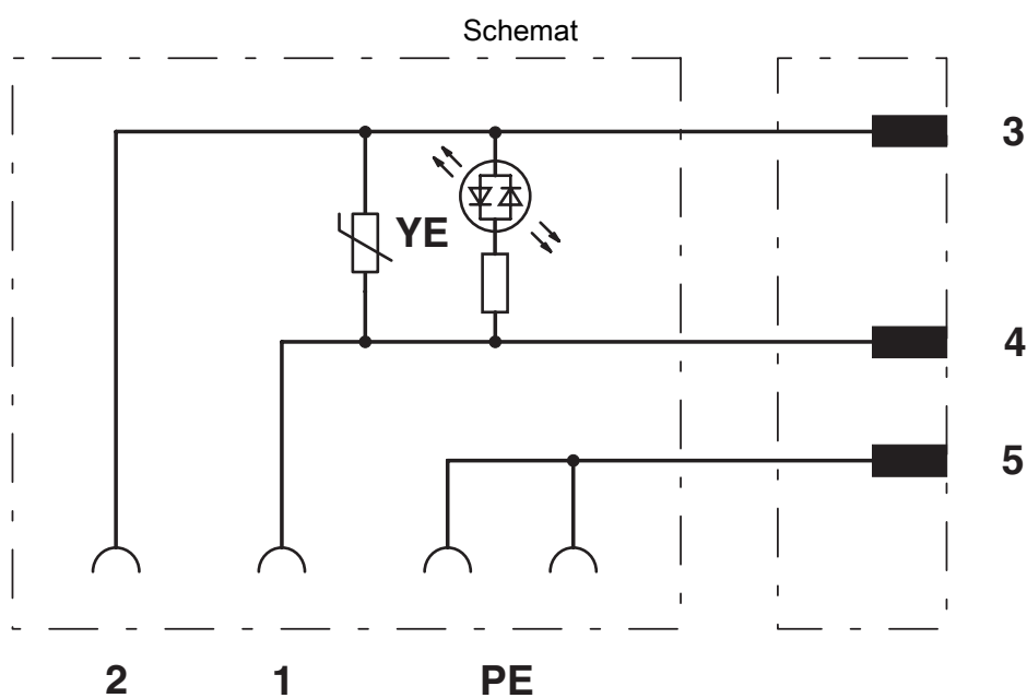
Układ styków wtyk M12, 3-biegunowy, wtyk zaworowy
