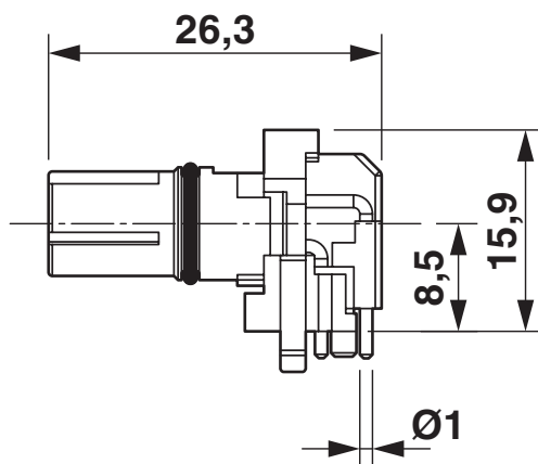
Rysunek wymiarowy
