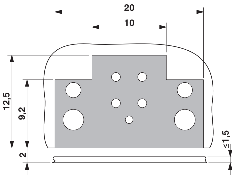
Rysunek wymiarowy
