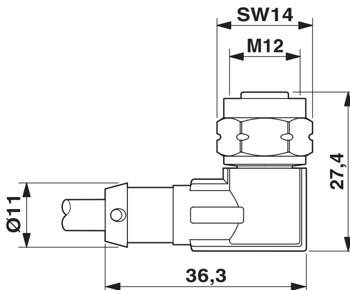
Rysunek wymiarowy
