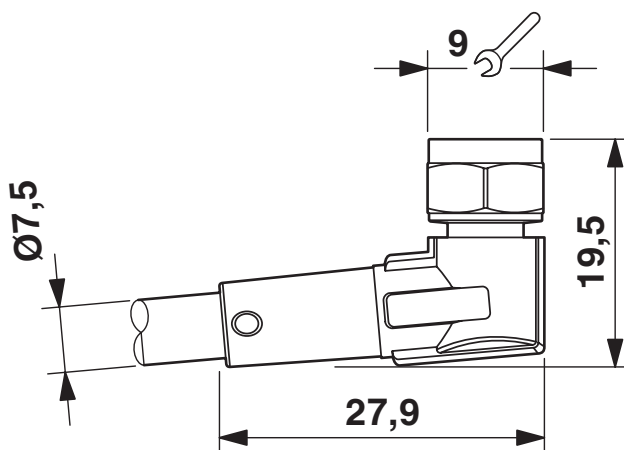
Rysunek wymiarowy
