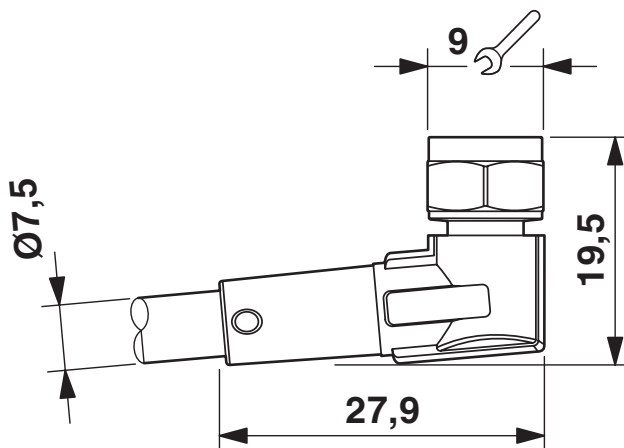
Rysunek wymiarowy
