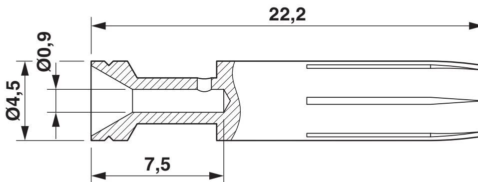
Rysunek wymiarowy
