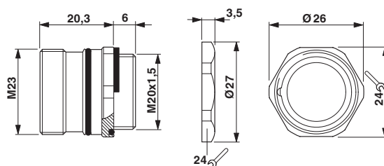
Rysunek wymiarowy
