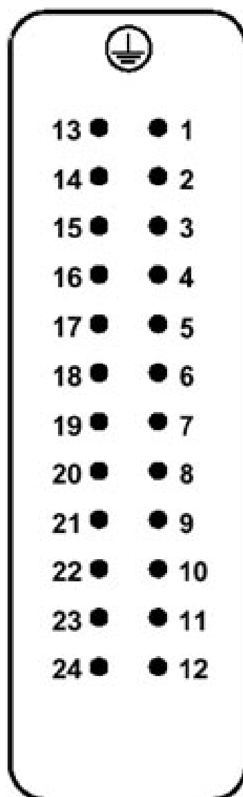
Rysunek schematyczny
