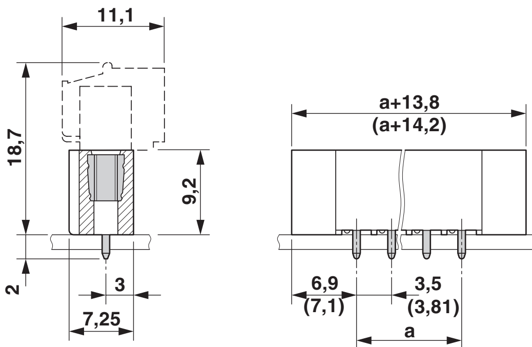
Rysunek wymiarowy
