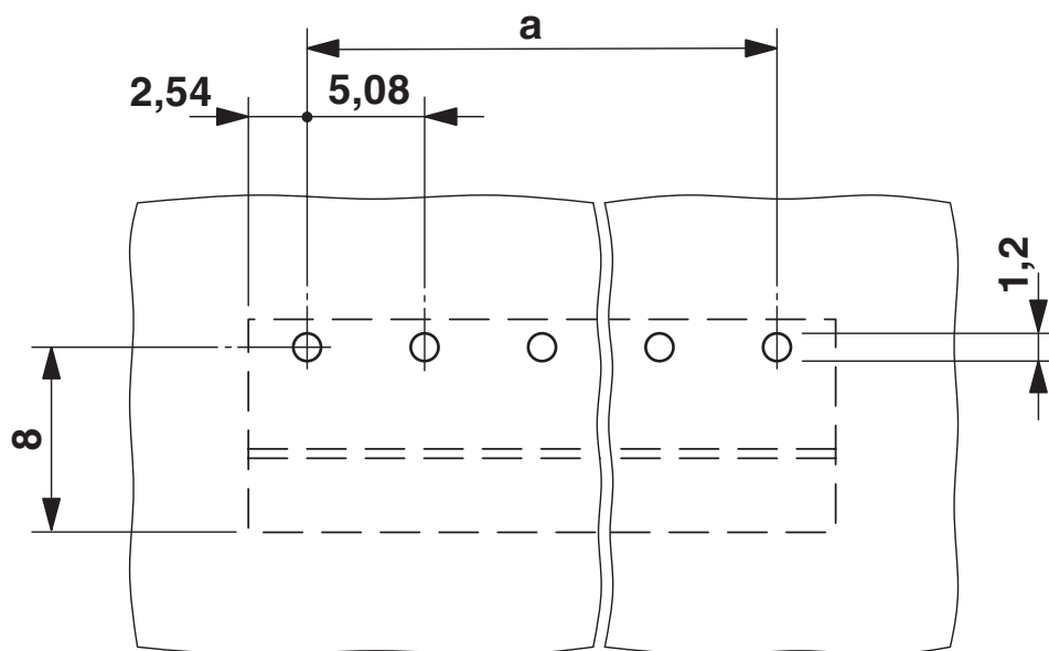
Otworowanie/geometria płytek lutowiczych
