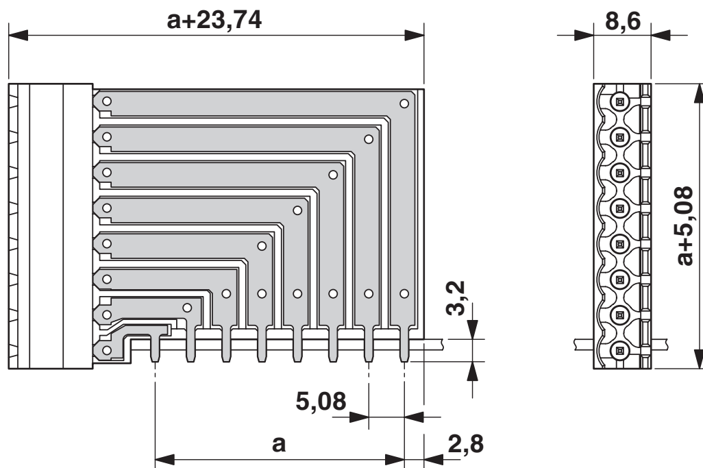
Rysunek wymiarowy
