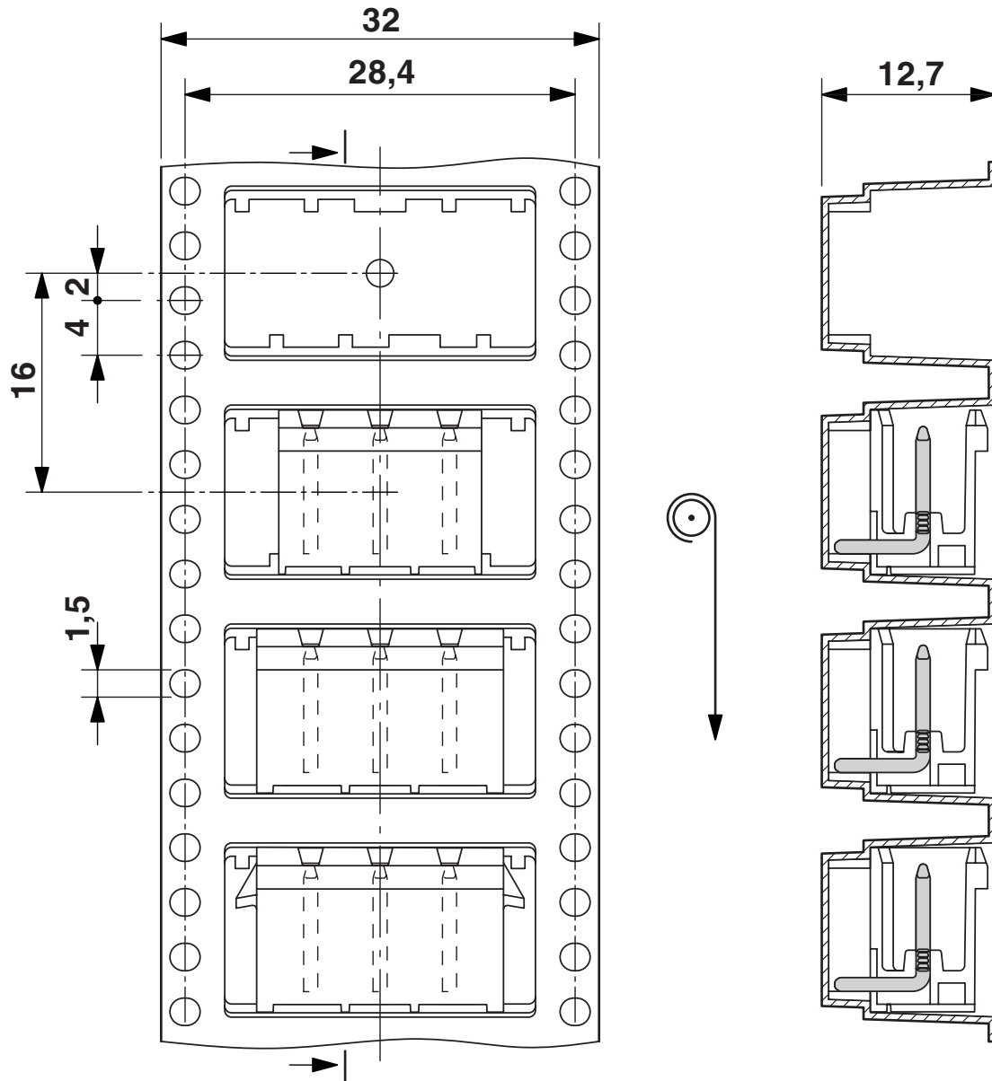
Rysunek wymiarowy
