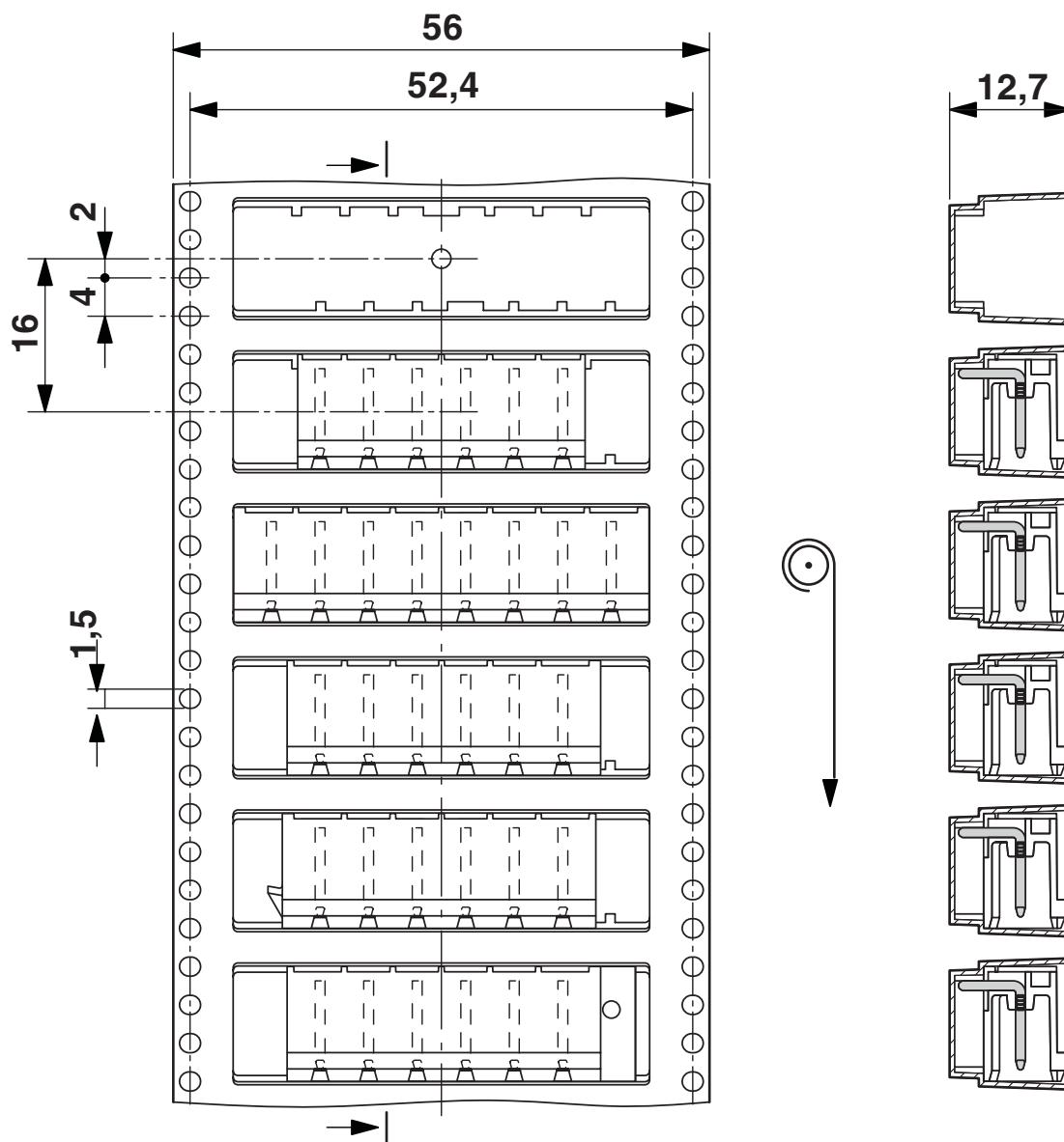
Rysunek wymiarowy
