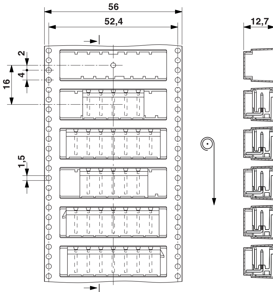
Rysunek wymiarowy
