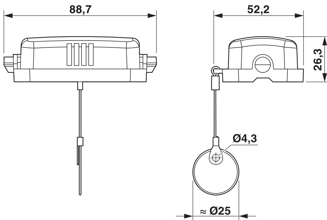
Rysunek wymiarowy
