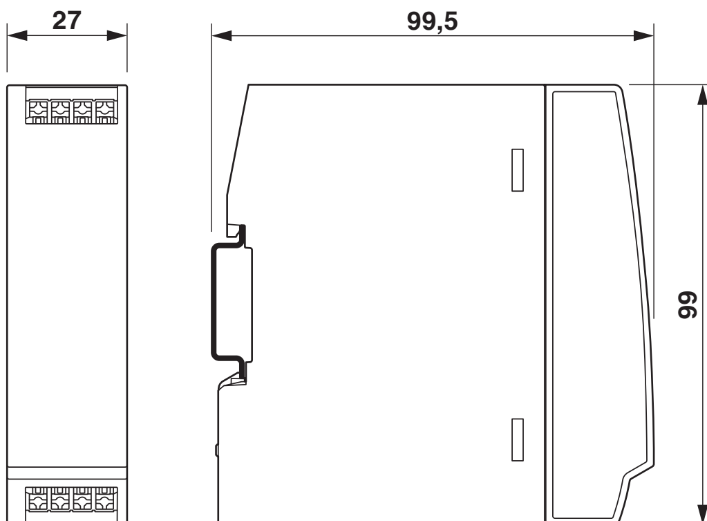
Rysunek wymiarowy
