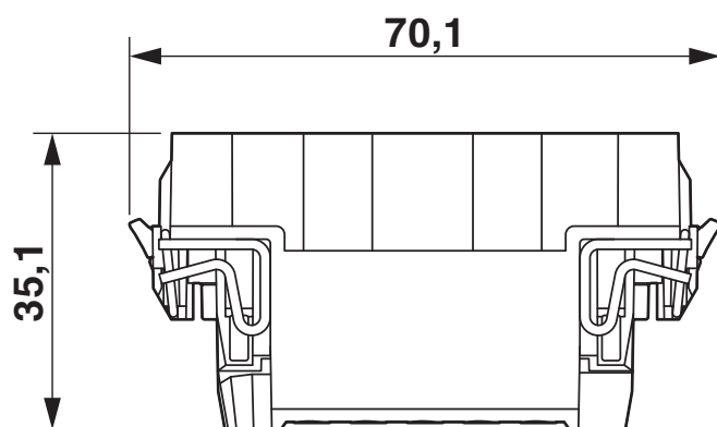
Rysunek wymiarowy
