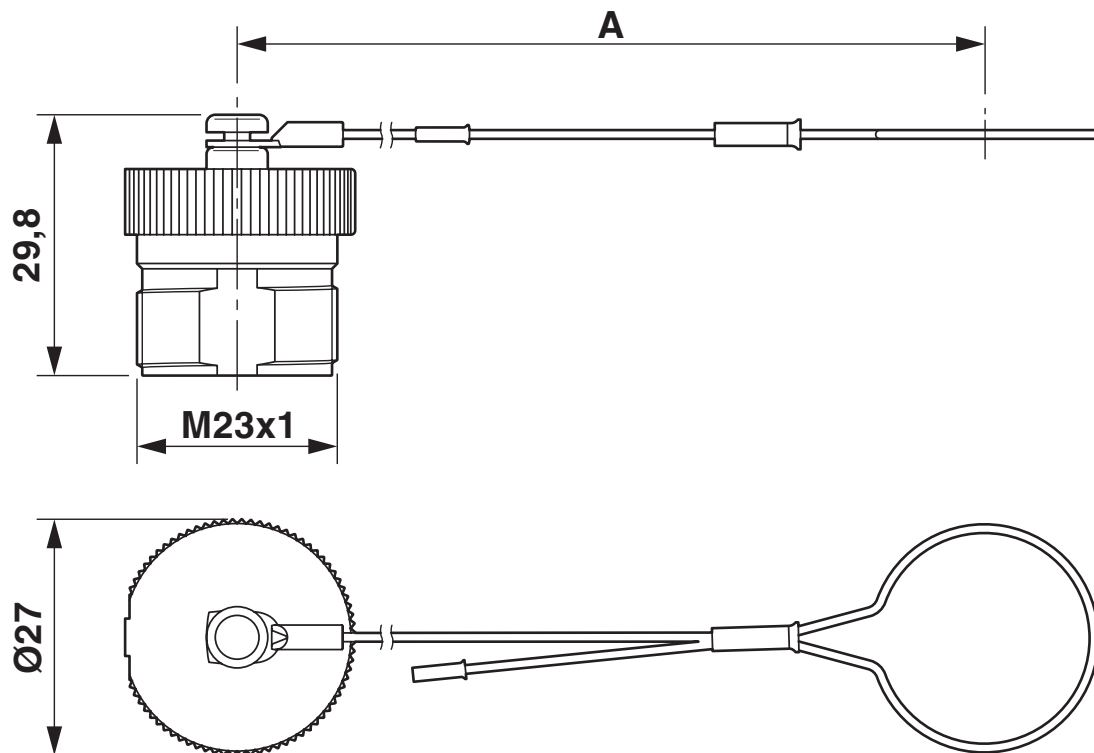
Rysunek wymiarowy
