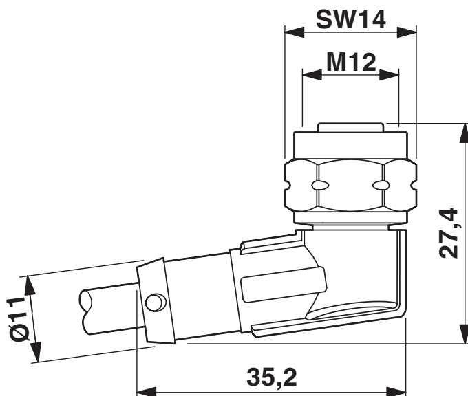
Rysunek wymiarowy
