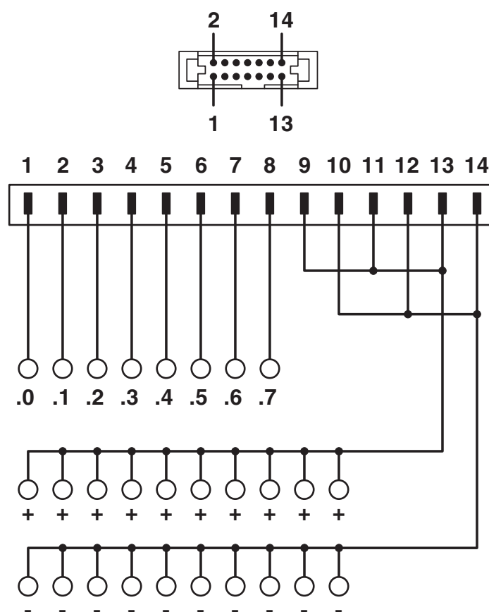
Schemat
