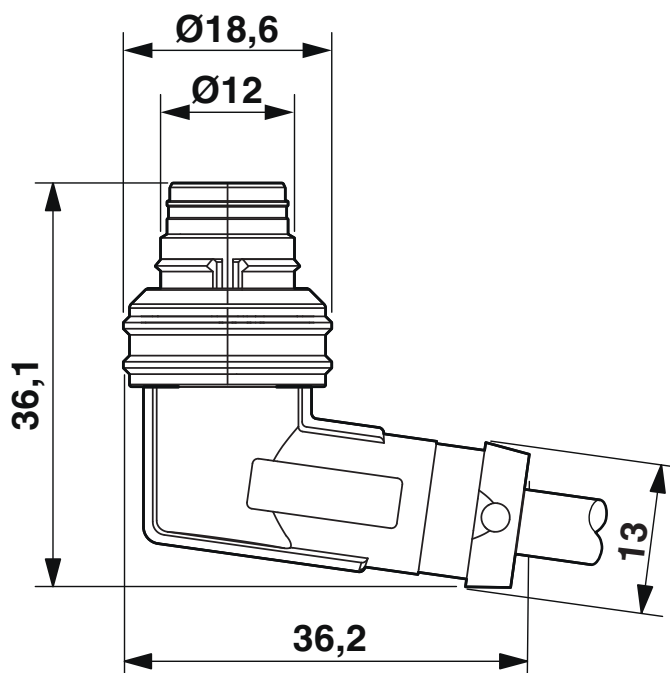
Rysunek wymiarowy
