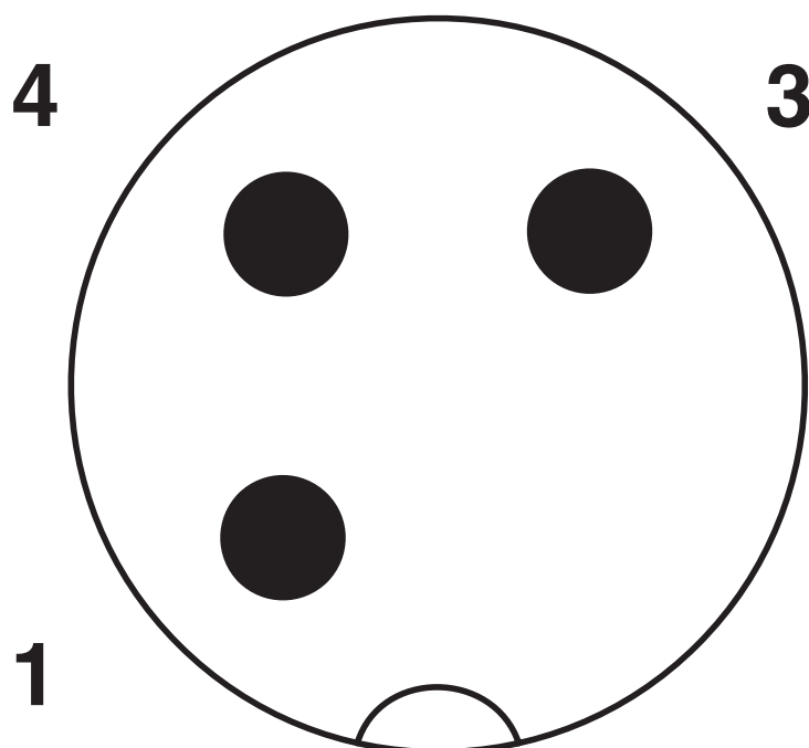
Rysunek schematyczny
