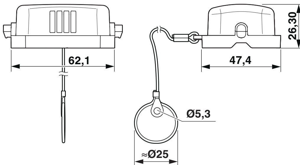
Rysunek wymiarowy
