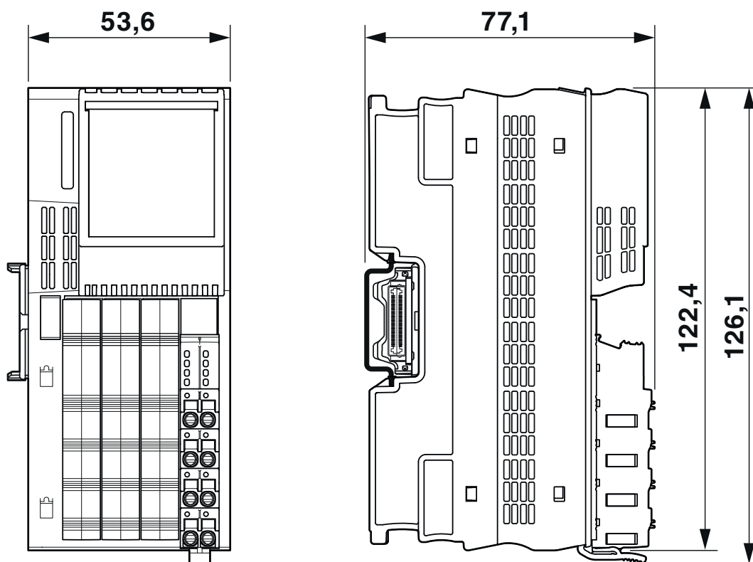
Rysunek wymiarowy
