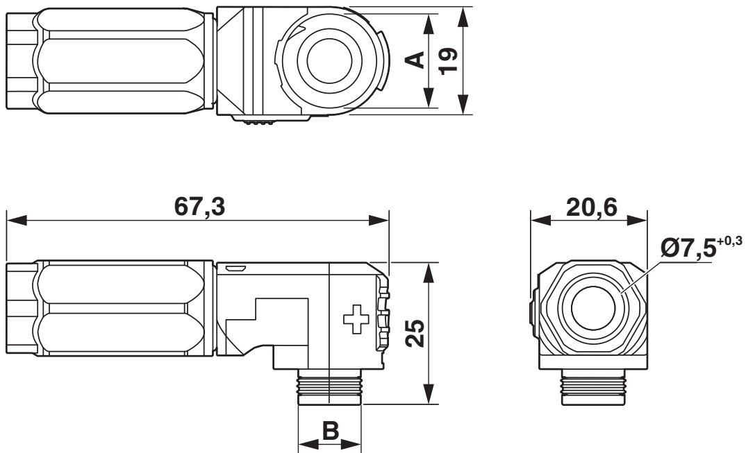
Rysunek wymiarowy
