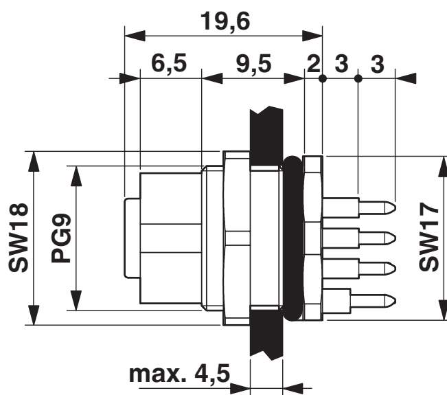
Rysunek wymiarowy
