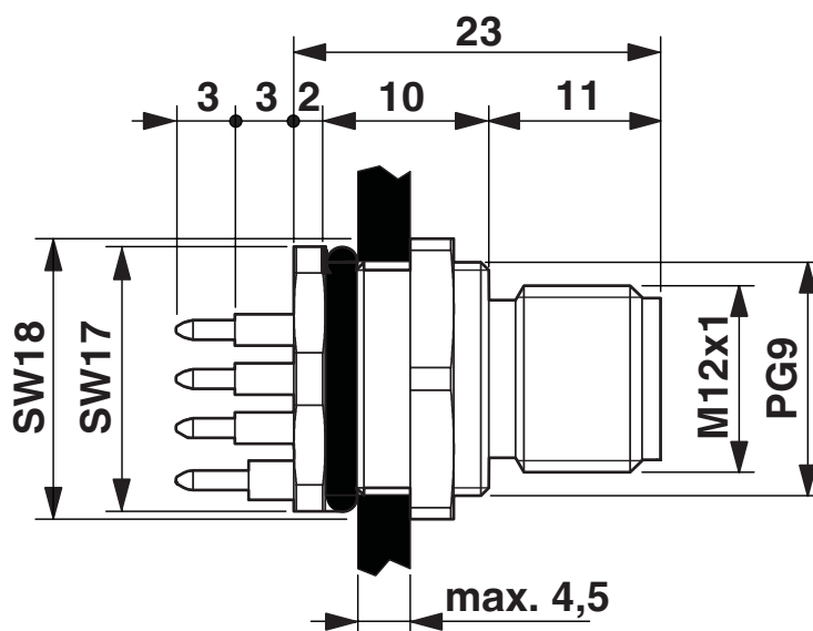
Rysunek wymiarowy
