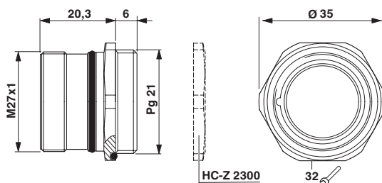
Rysunek wymiarowy
