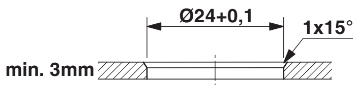
Rysunek wymiarowy
