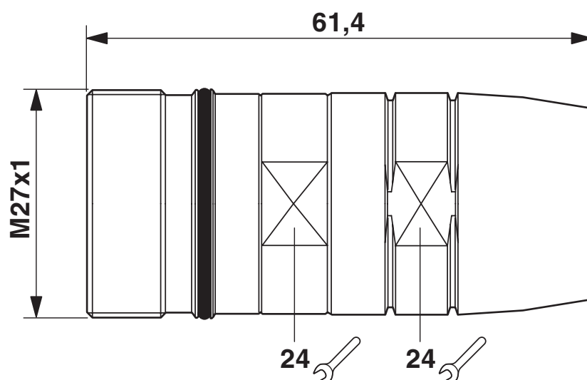
Rysunek wymiarowy
