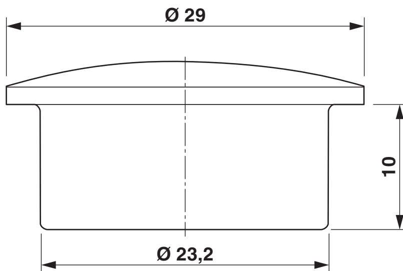
Rysunek wymiarowy
