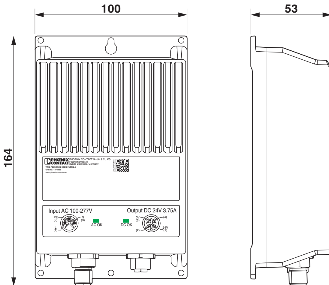
Rysunek wymiarowy
