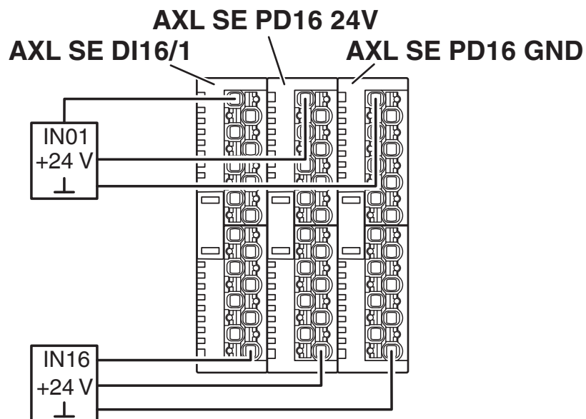
rysunek złączy
