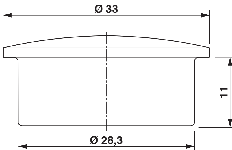
Rysunek wymiarowy
