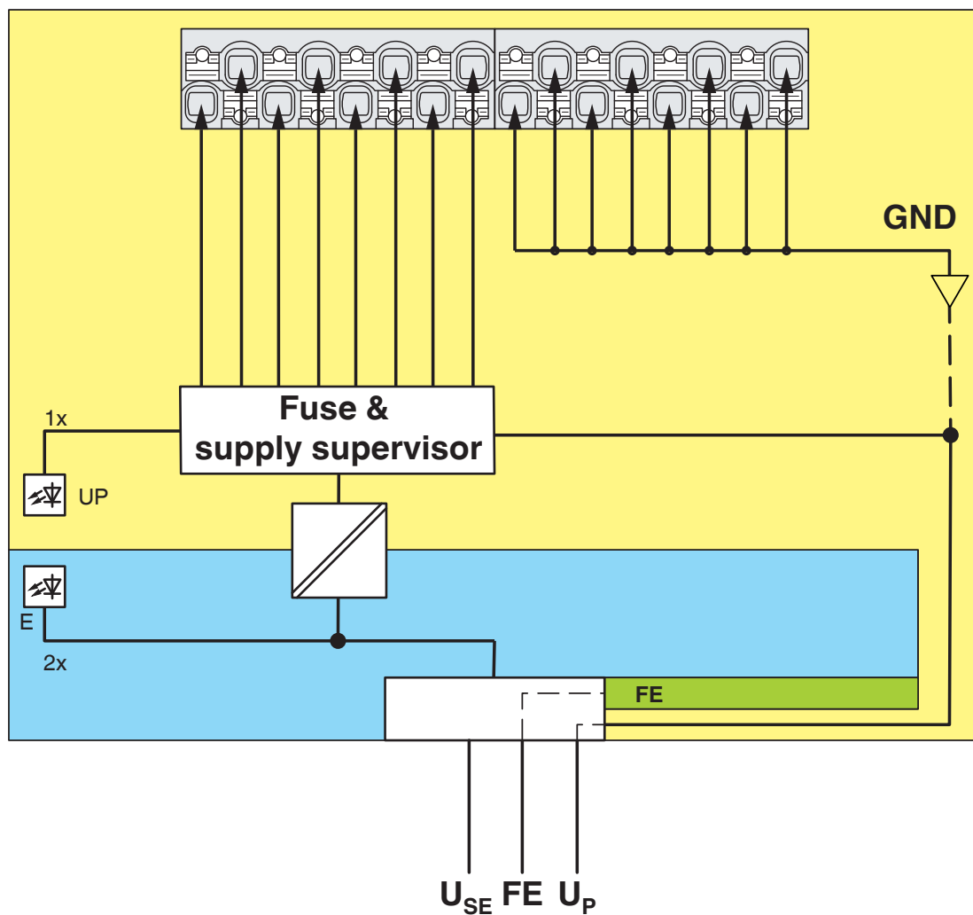
Schemat blokowy
