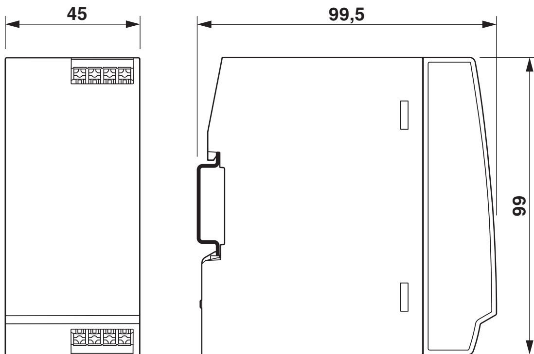
Rysunek wymiarowy
