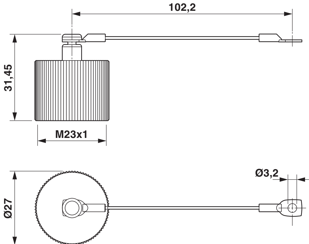
Rysunek wymiarowy
