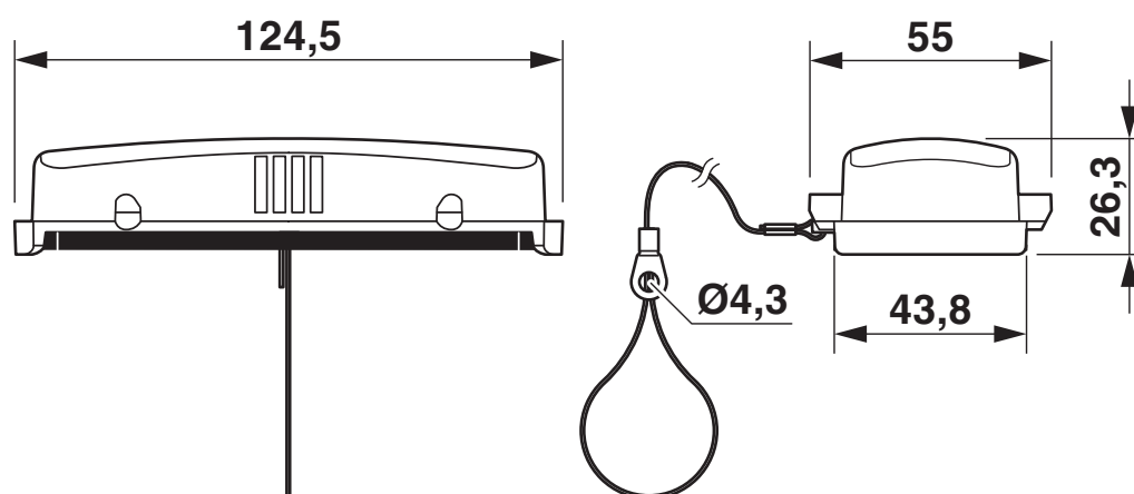
Rysunek wymiarowy
